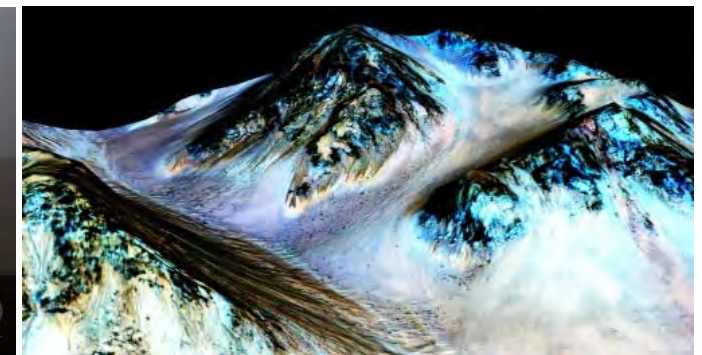
液体の水が流れている証拠発見 (2015年9月29日)
