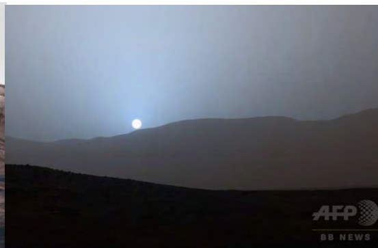
火星の青い夕焼け (2015年5月14日)
